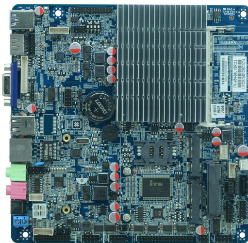
图一： ITX-M50 主板正面图
