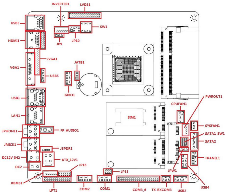
ITX-M50 接口位置图
